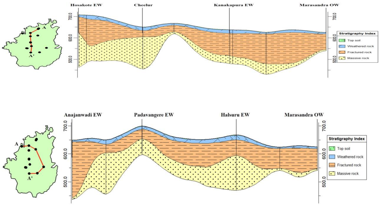
Fig.13a:2-D Aquifer disposition
